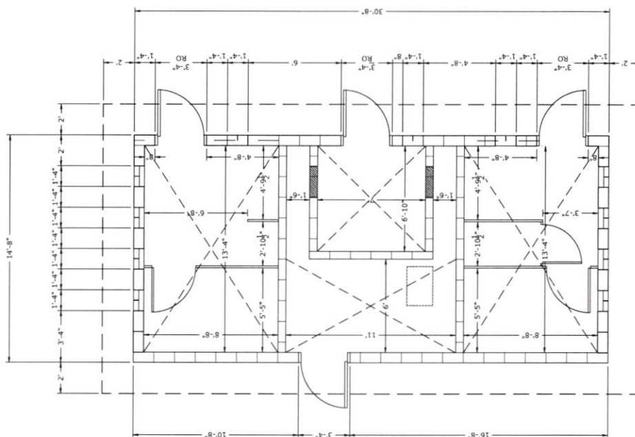
FLOOR PLAN 22x34 SCALE: 3/8" = 1'-0" 11x17 SCALE: 3/16" = 1'-0"
